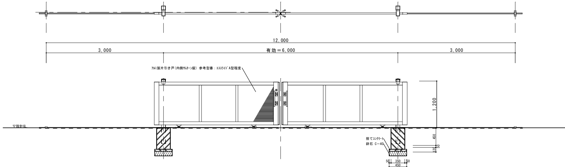
出入口門扉②詳細図 S=1/30
