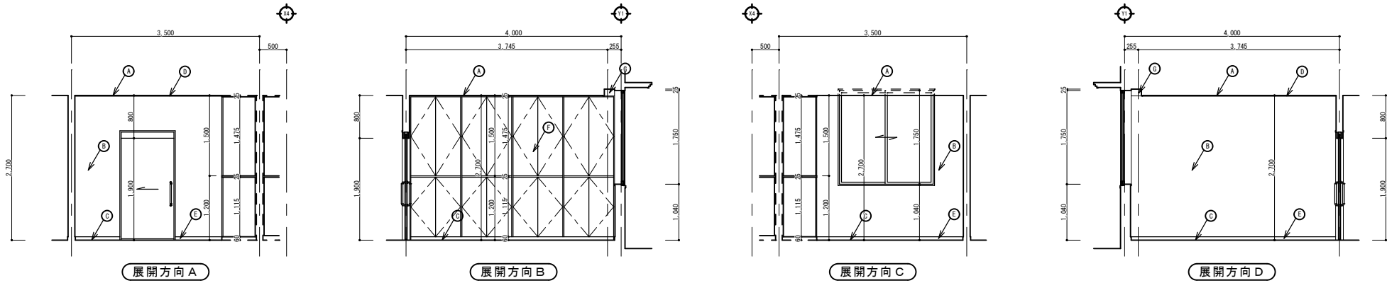
ケアルーム1展開図 S=1/50
