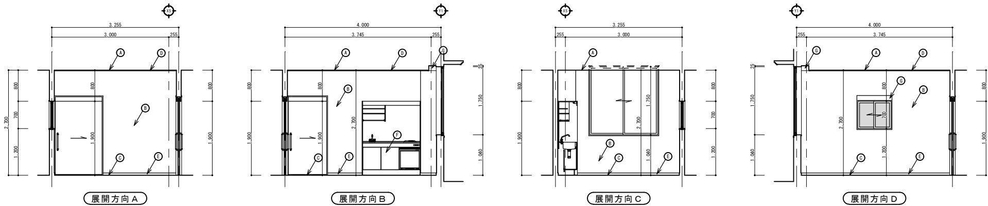
医務室展開図 S=1/50
