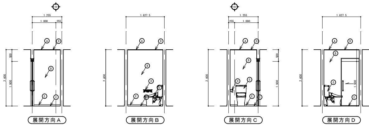
従業員用トイレ男展開図 S=1/50
