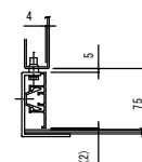
U幅木詳細 (1 / 5)
