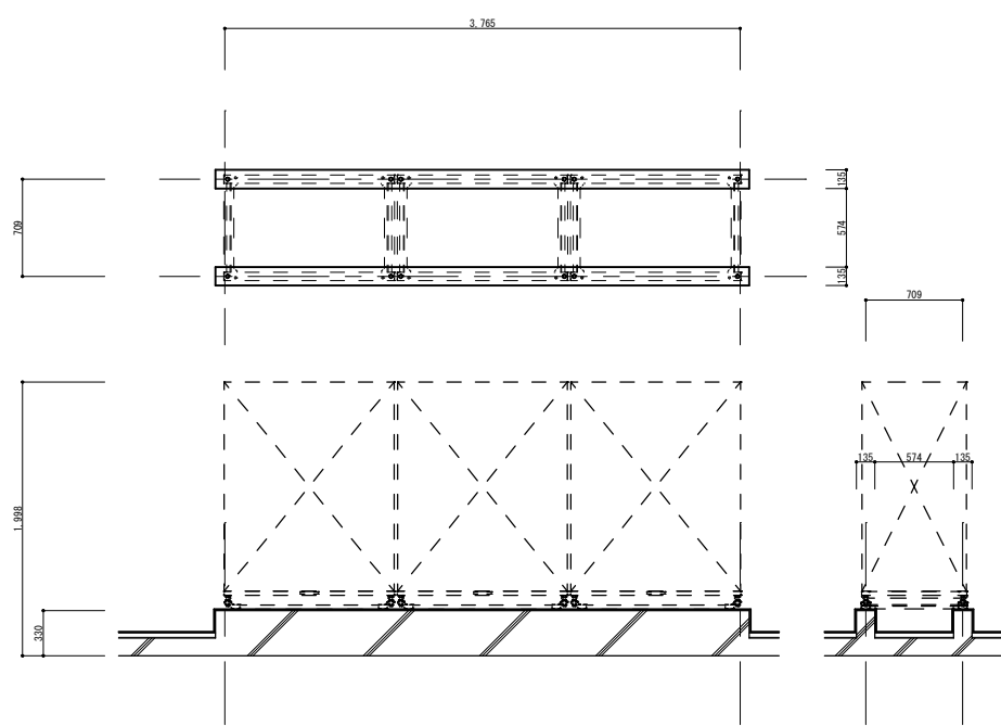
室外機架台基礎断面詳細図 S=1/30
