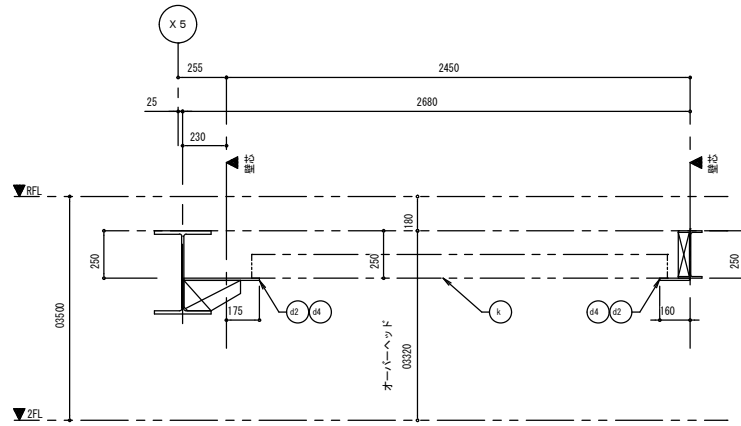
断面X-X
