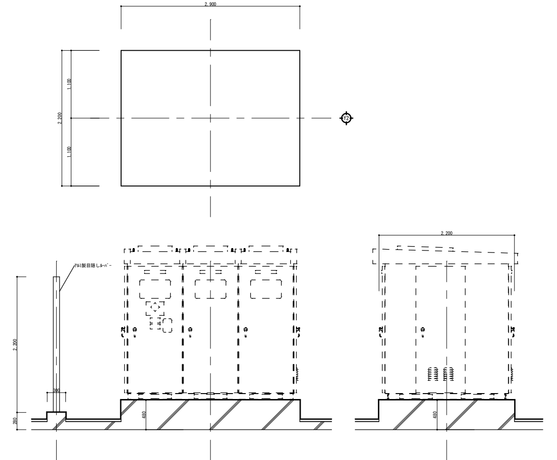
変電設備基礎断面詳細図 S=1/30
