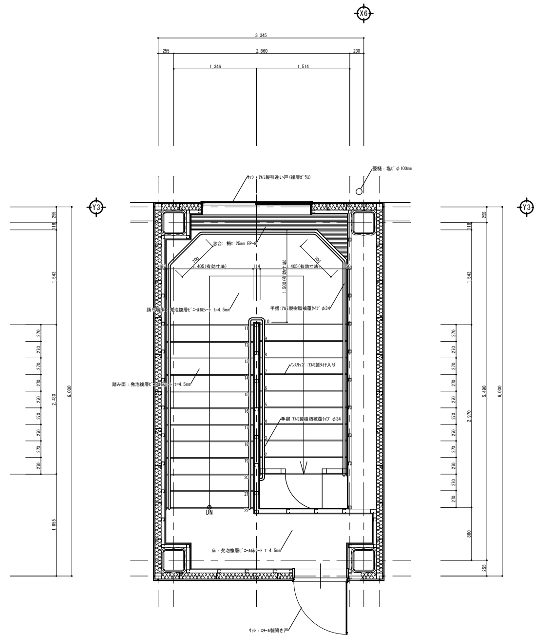
PH階階段平面詳細図 S=1/30
