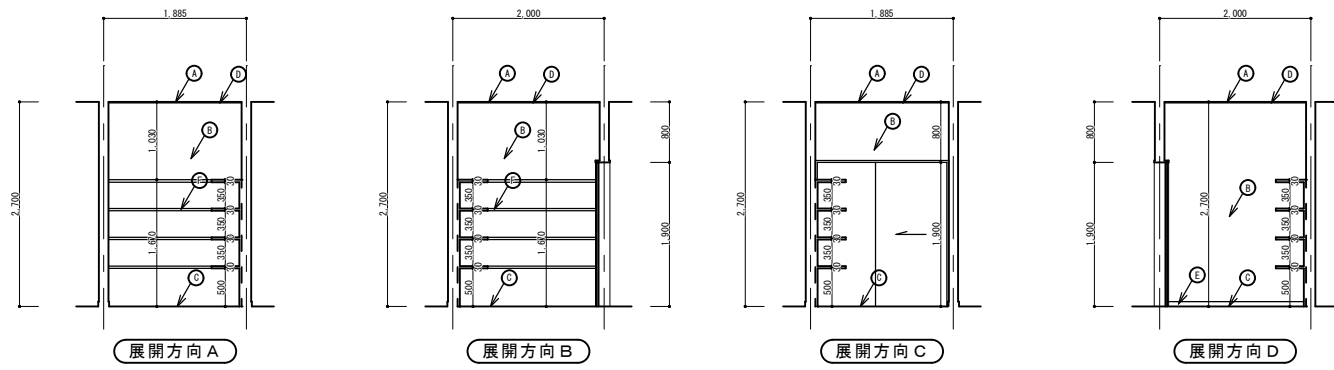
食品庫展開図 S=1/50
