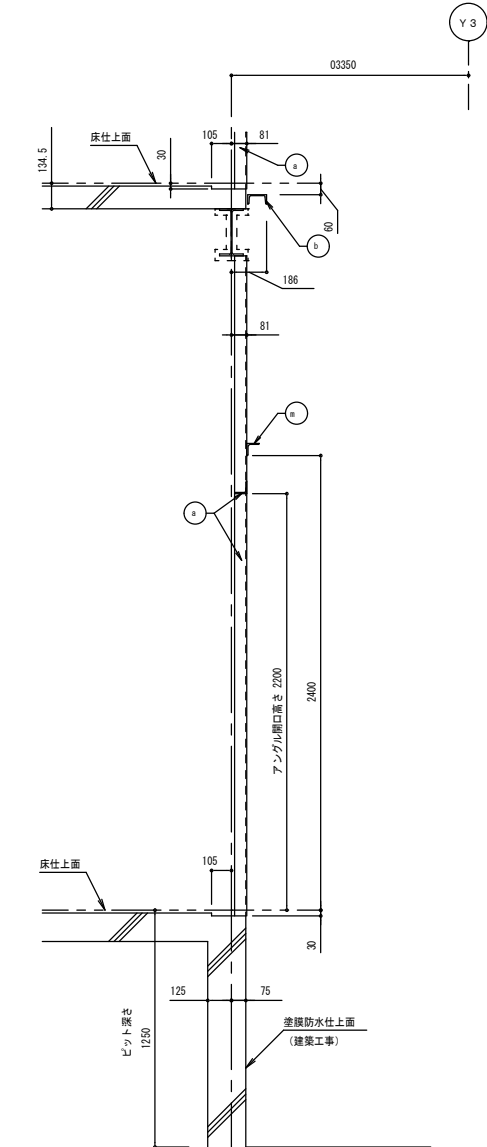
X-X 断面
