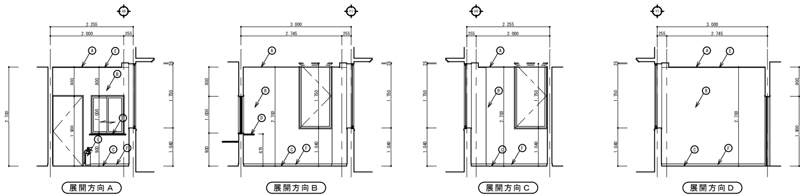
管理室展開図 S=1/50
