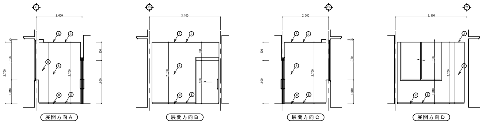
職員用更衣室展開図 S=1/50
