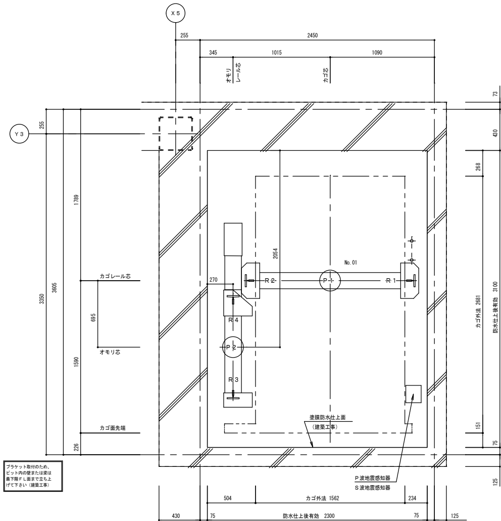
昇降路平面図 (1/20) (ビット)
