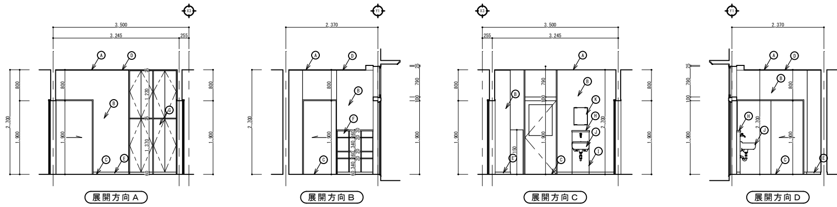
検品室展開図 S=1/50
