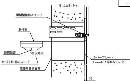
矢視A-A
