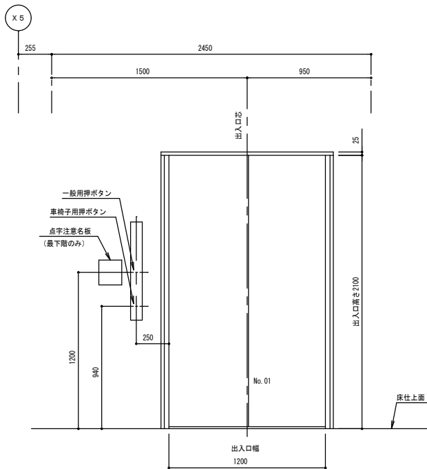
乗場正面図 (1/20)
