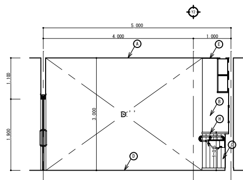
展開方向 D'
