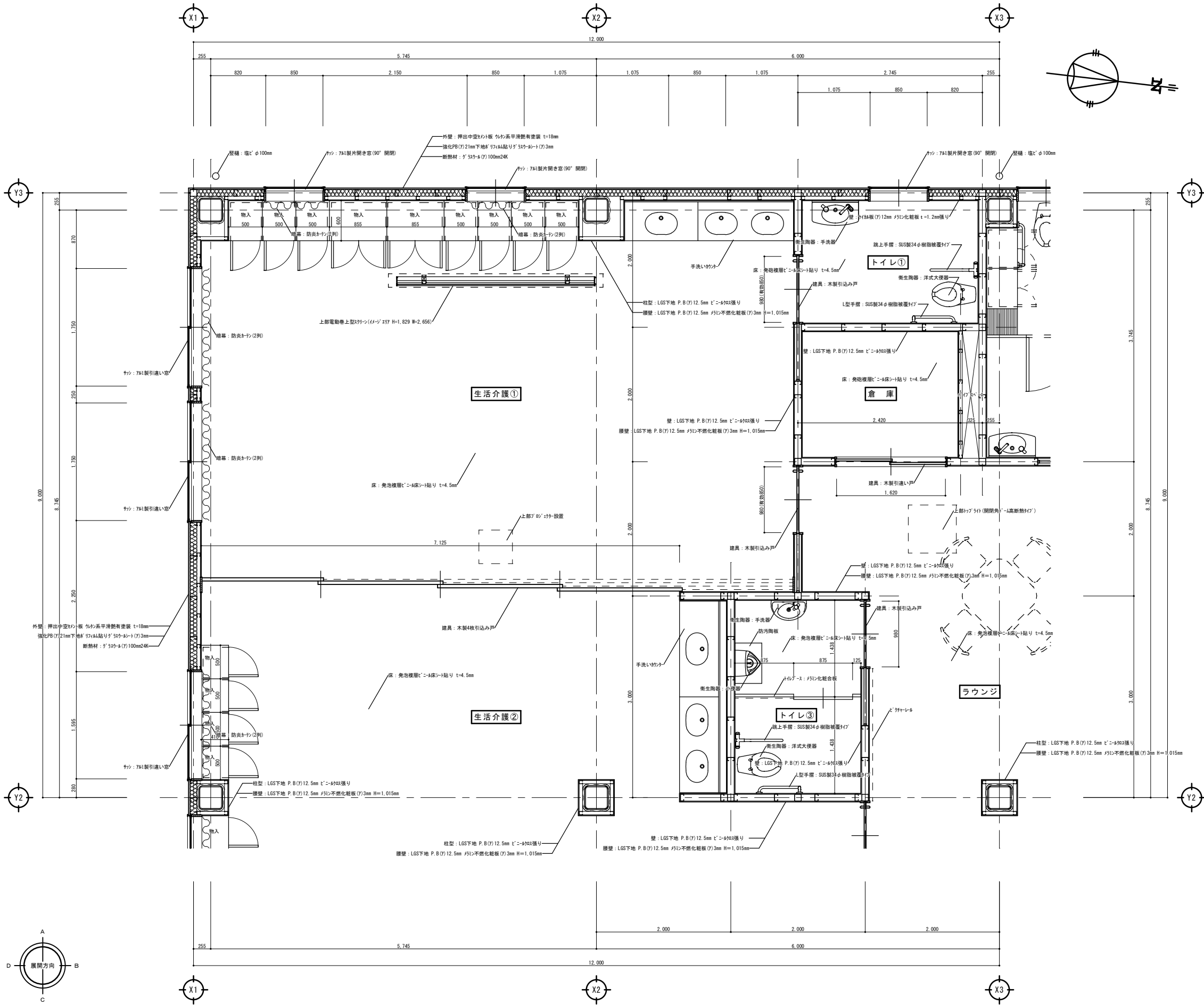
2 階平面詳細図－6 S=1/30
