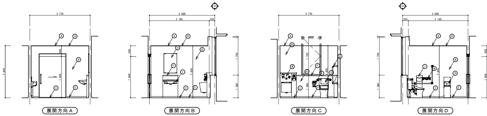
多機能トイレ展開図 S=1/50
