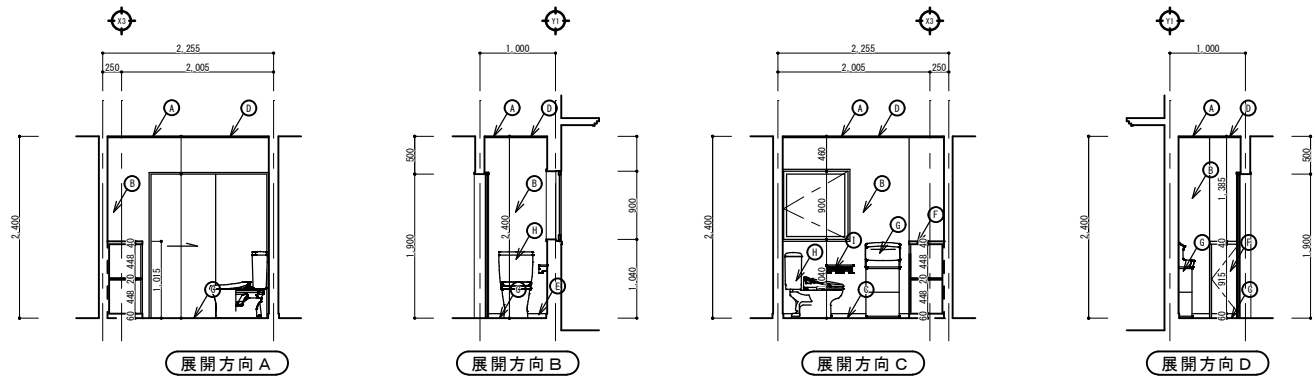
従業員用トイレ展開図 S=1/50
