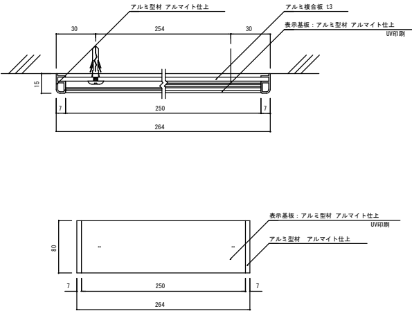
室名札詳細図 S=1/2
