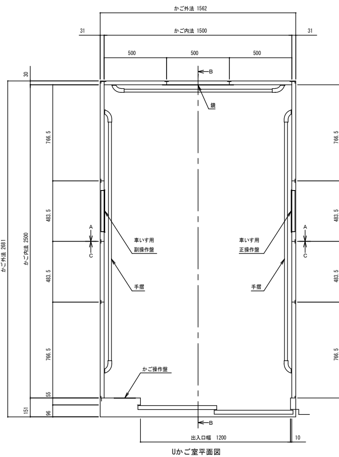
Uかご室平面図
