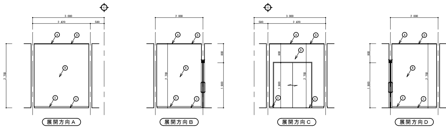
倉庫展開図 S=1/50
