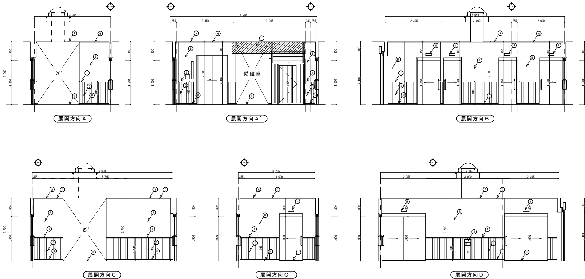
ホール展開図 S=1/50
