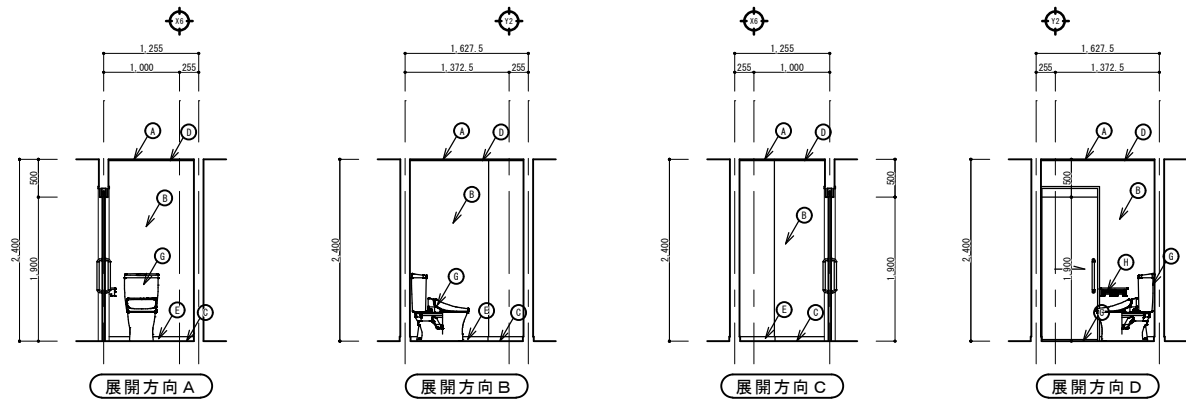
従業員用トイレ女展開図 S=1/50
