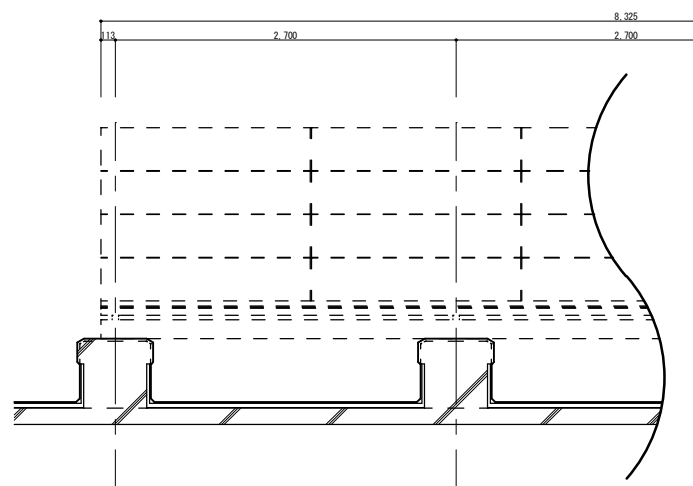
太陽光発電基礎断面詳細図 S=1/30
