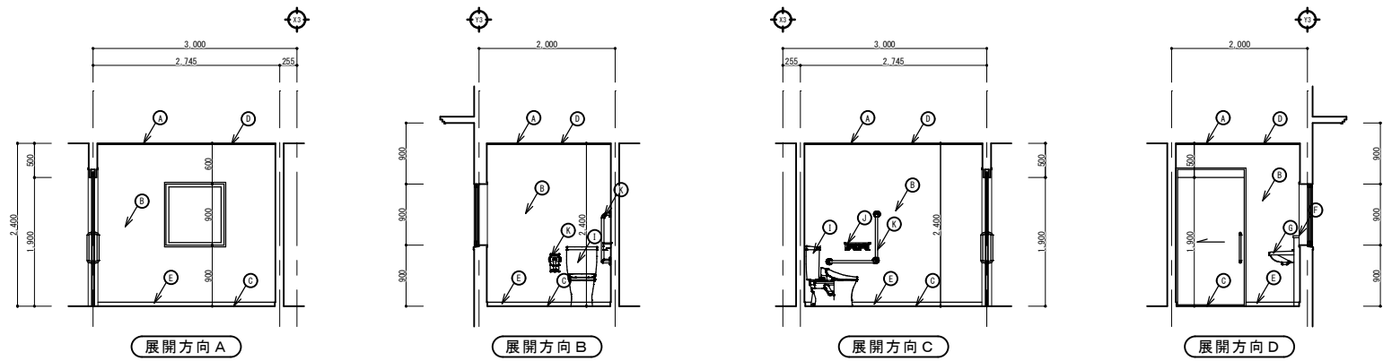
トイレ1展開図 S=1/50
