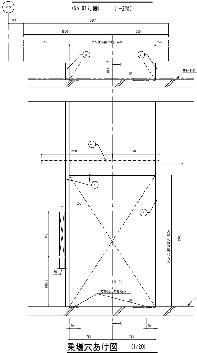
(No. 01号機) (1-2階)
