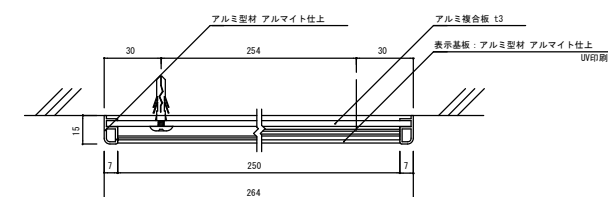
室名札詳細図 S=1/2
