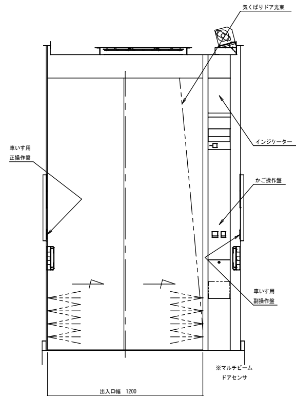
Uかご室正面図 (A-A断面)
