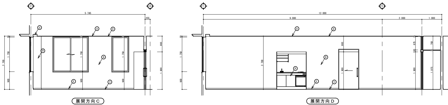
事務室2展開図 S=1/50
