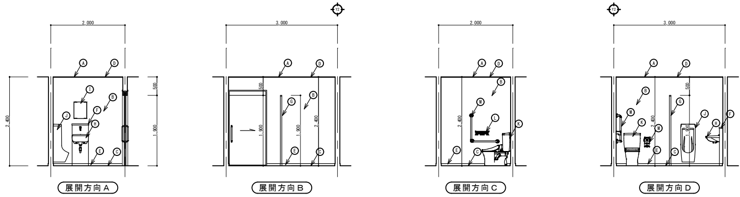
トイレ3展開図 S=1/50
