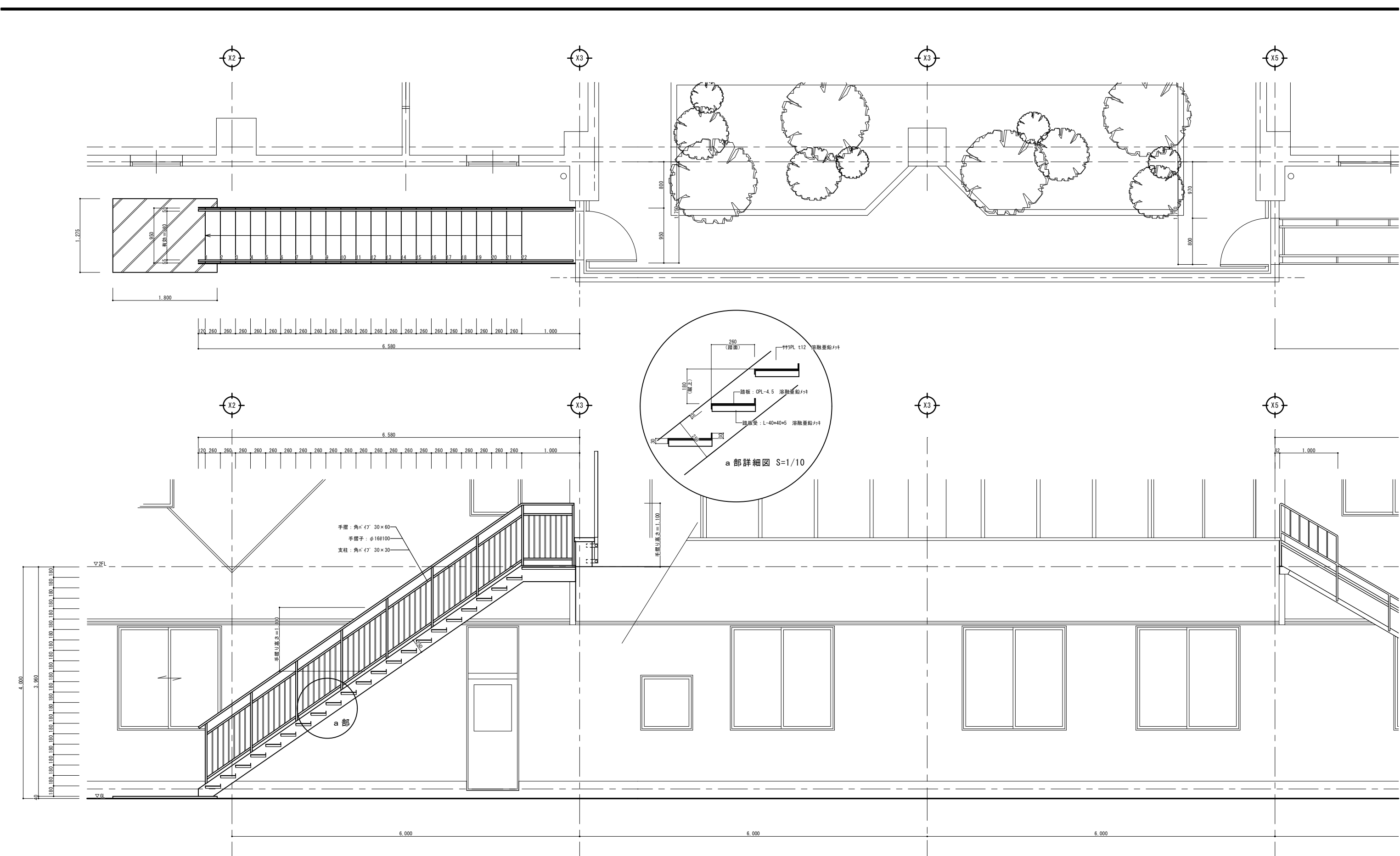
屋外階段詳細図 S=1/30
