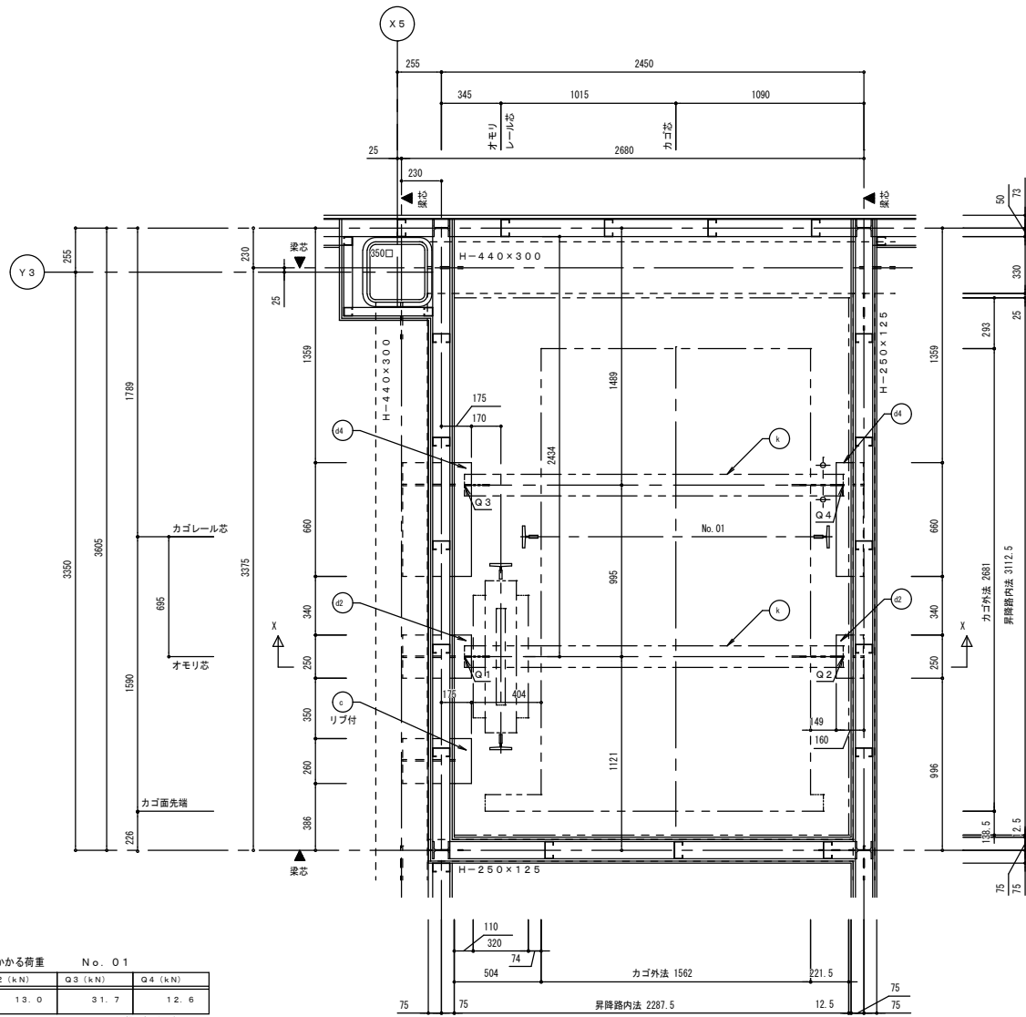
昇降路平面図 (1/20) (頂部)
