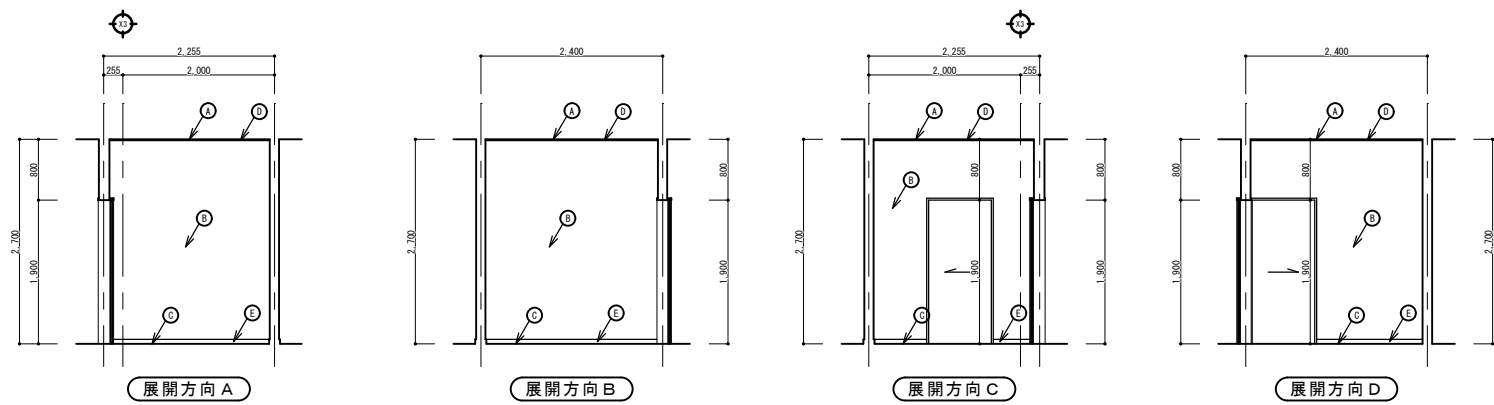
更衣室展開図 S=1/50
