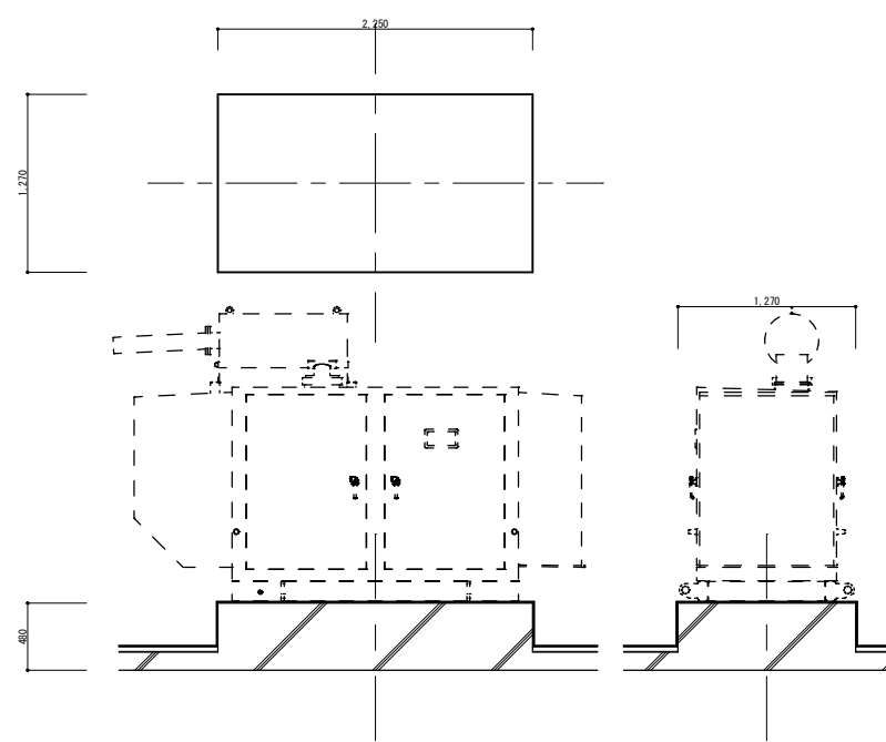
自家発電設備基礎断面詳細図 S=1/30
