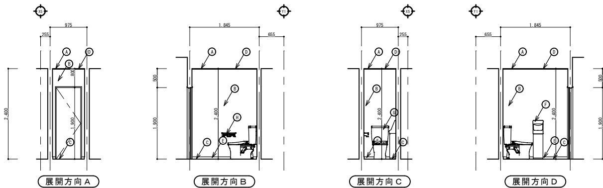
従業員用トイレ展開図 S=1/50
