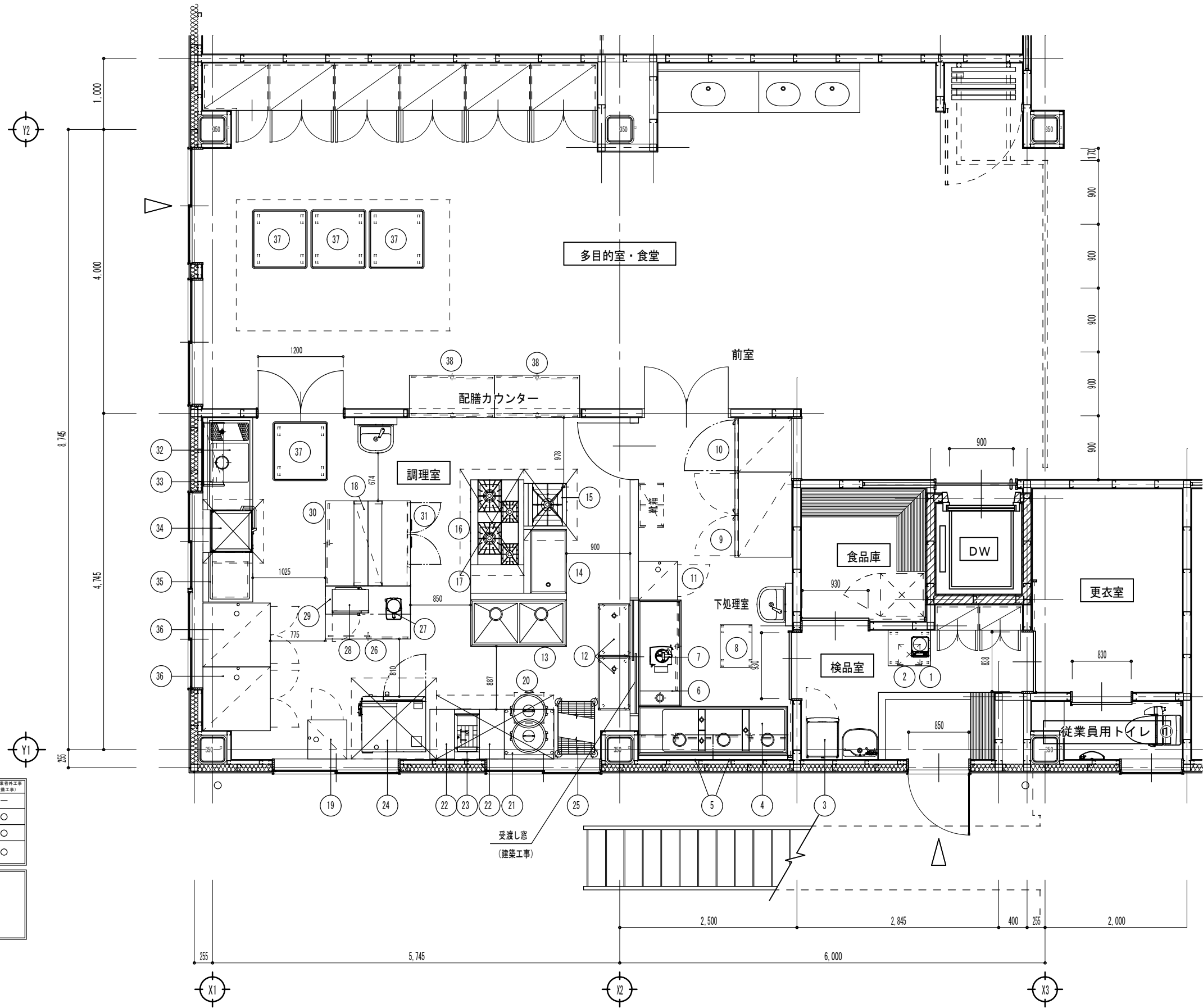
厨房平面詳細図 S=1/30
