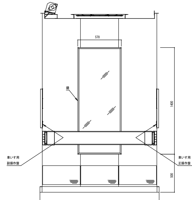
Uかご室背面図 (C-C断面)
