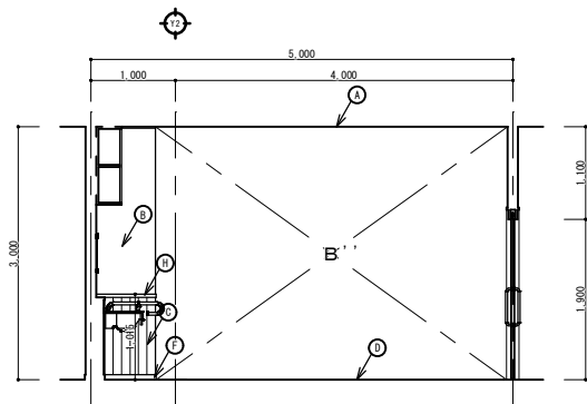
展開方向 B'
