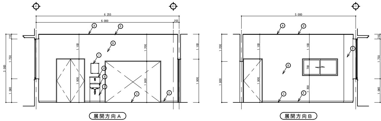
下処理室展開図 S=1/50
