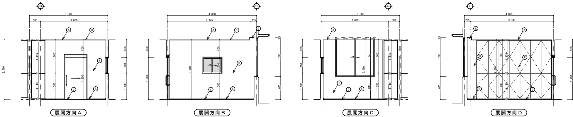
ケアルーム2展開図 S=1/50
