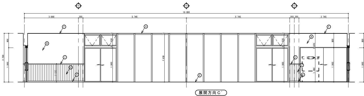
ラウンジ展開図 S=1/50
