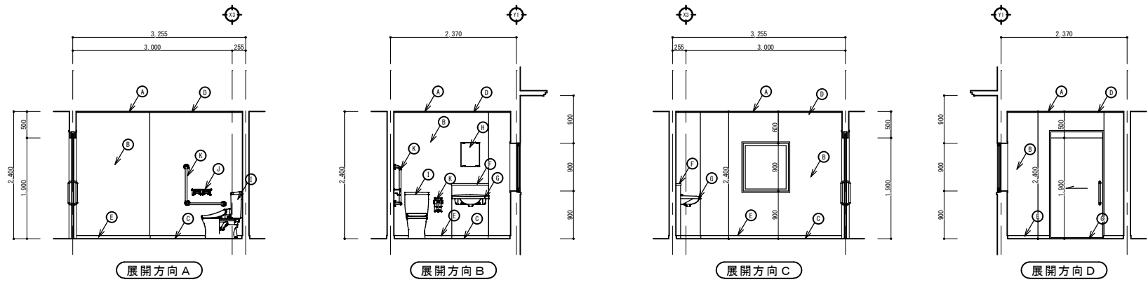
トイレ2展開図 S=1/50
