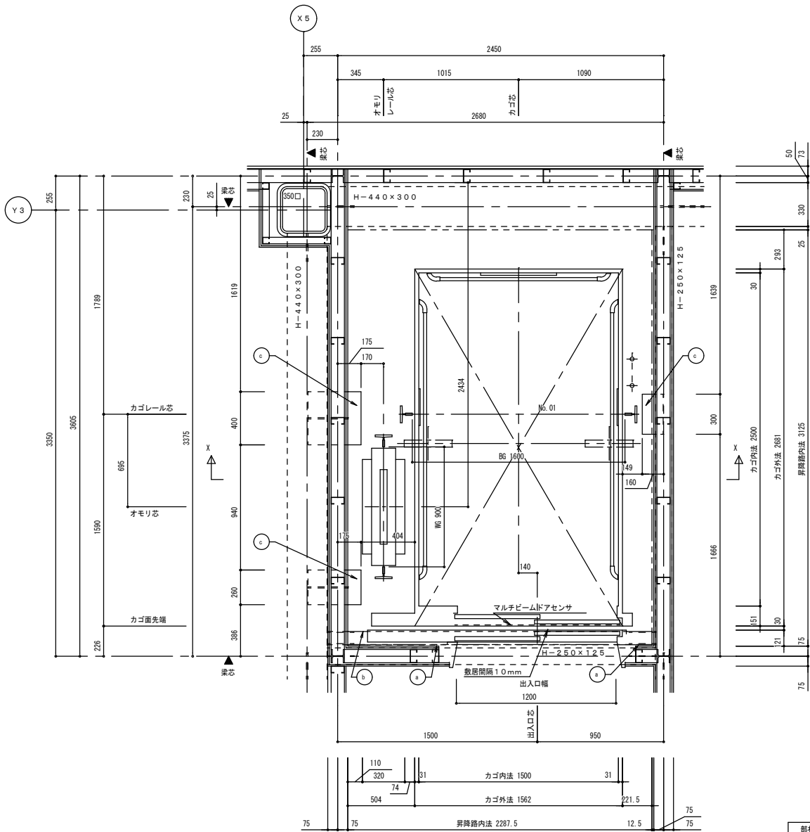
昇降路平面図 (1/20) (2階)
