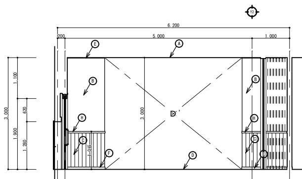
展開方向 D
