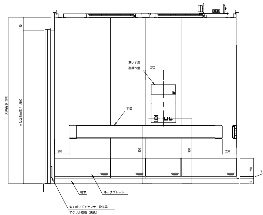
Uかご室側面図 (B-B断面)
