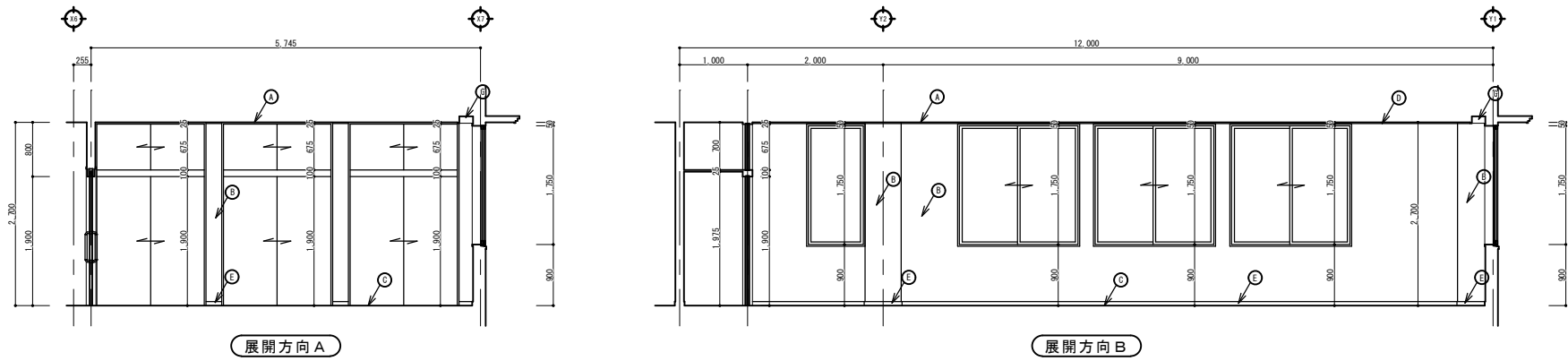
地域交流スペース展開図 S=1/50
