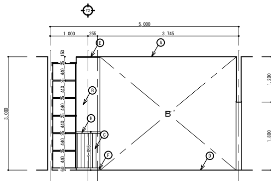
展開方向 B
