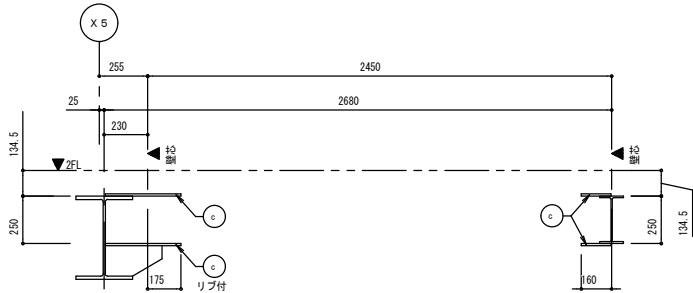
断面X-X
