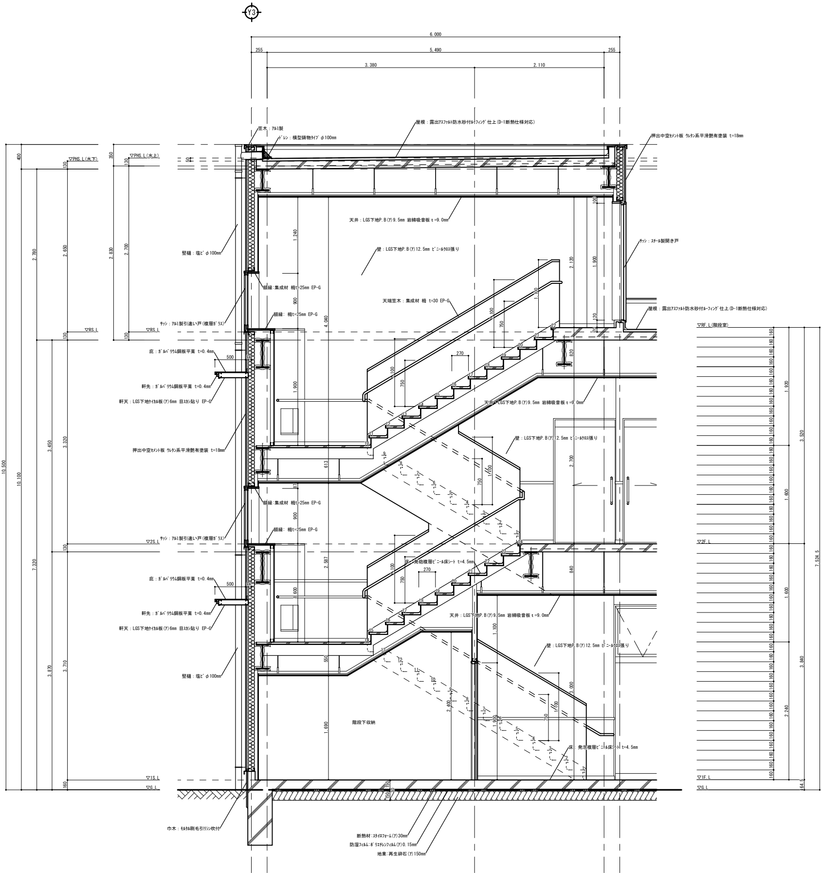
階段矩計図 S=1/30
