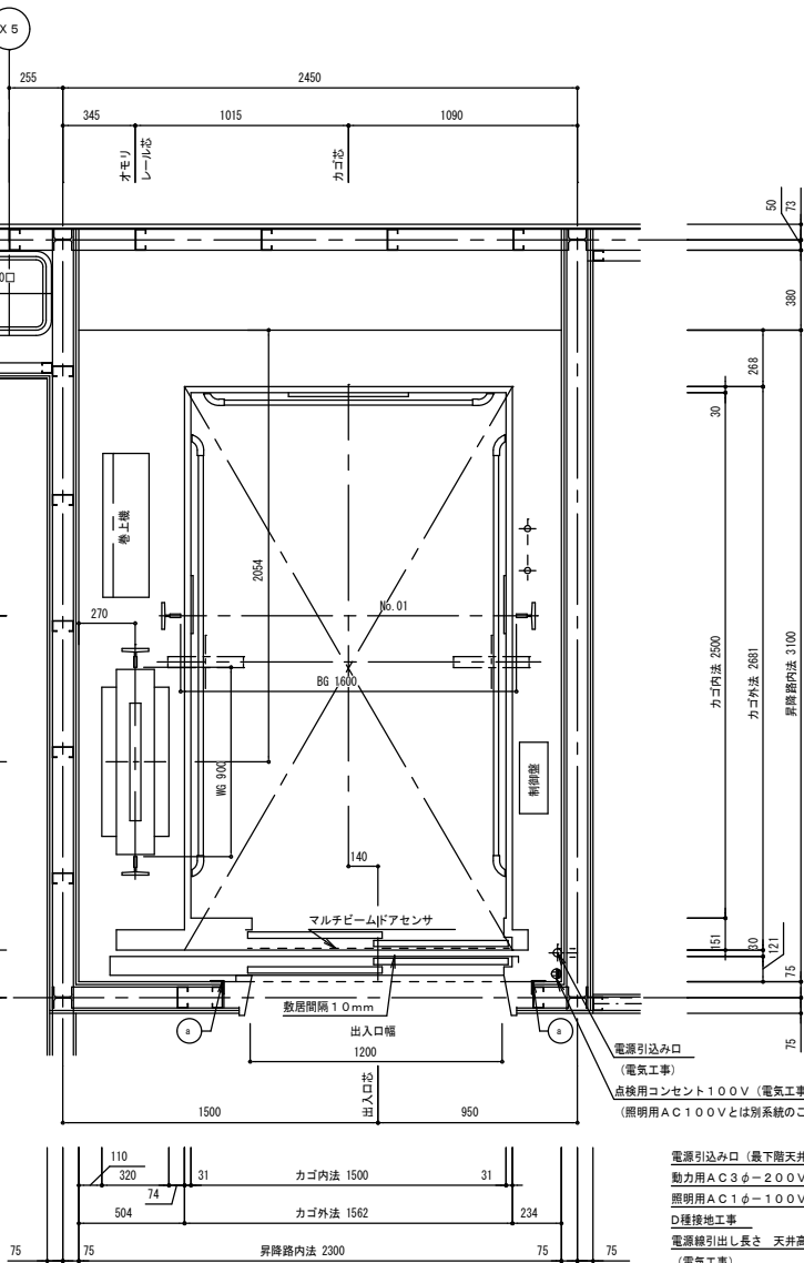
昇降路平面図 (1/20) (1階)
