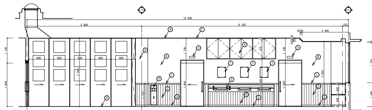
展開方向 D'
