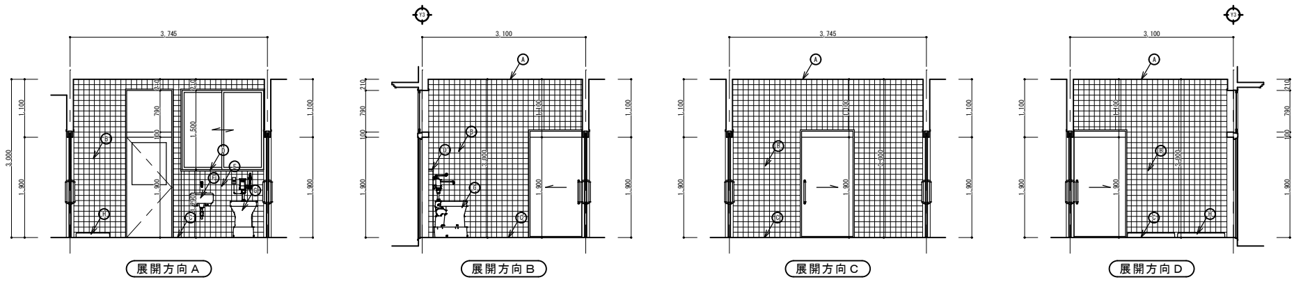
汚物・洗濯室展開図 S=1/50
